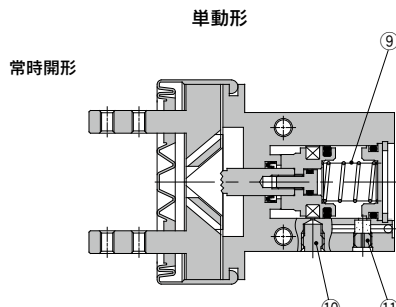
常時開形
